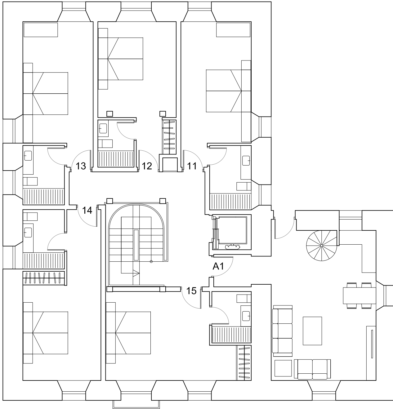
PLANTA PRIMERA
