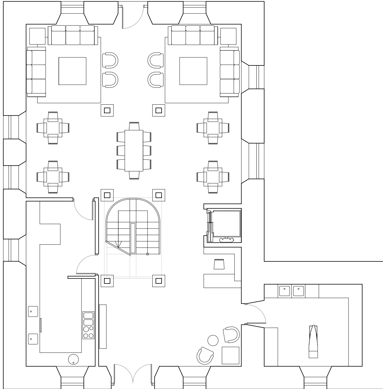
PLANTA BAJA
